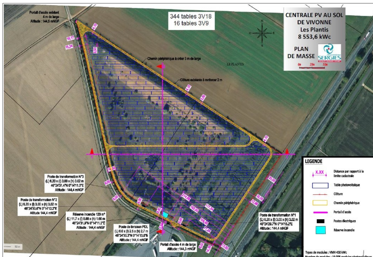
Plan masse du projet – extrait dossier de permis de construire
