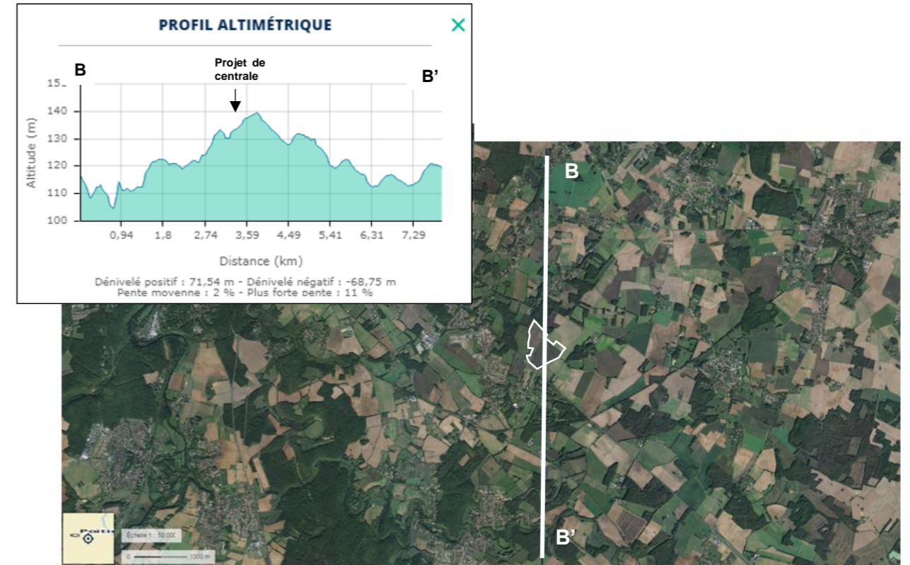
Figure I-5 : Profil altimétrique du site d'implantation de la future centrale photovoltaïque – Mignaloux-Beauvoir – Source Géoportail
