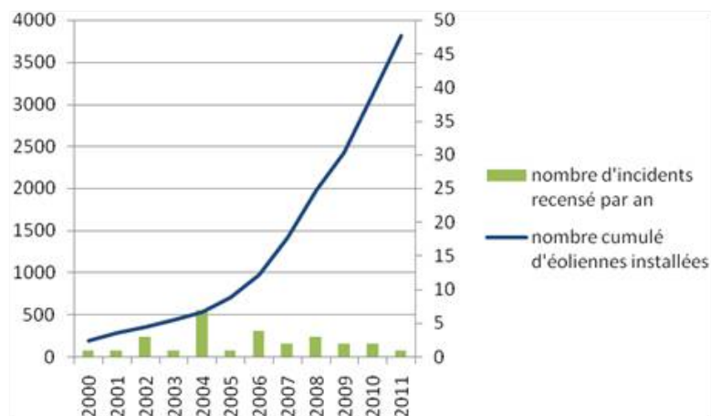
Figure 18 : Evolution du nombre d'incidents annuels en France et du nombre d'éoliennes installées
