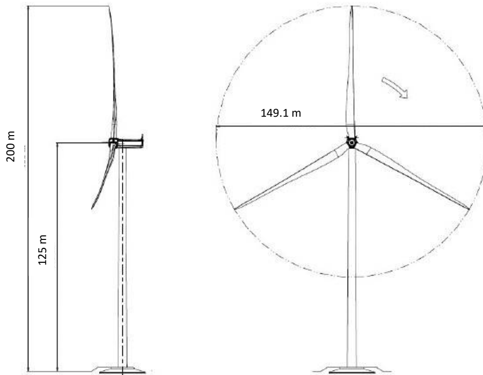
Figure 5 : Dessin d'élevation de l'éolienne N149- 4,5MW
