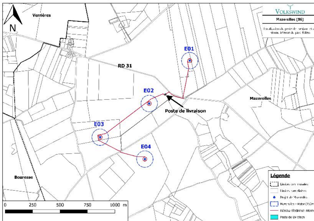
Carte 28 : Localisation du poste de livraison et réseau interne du parc éolien
