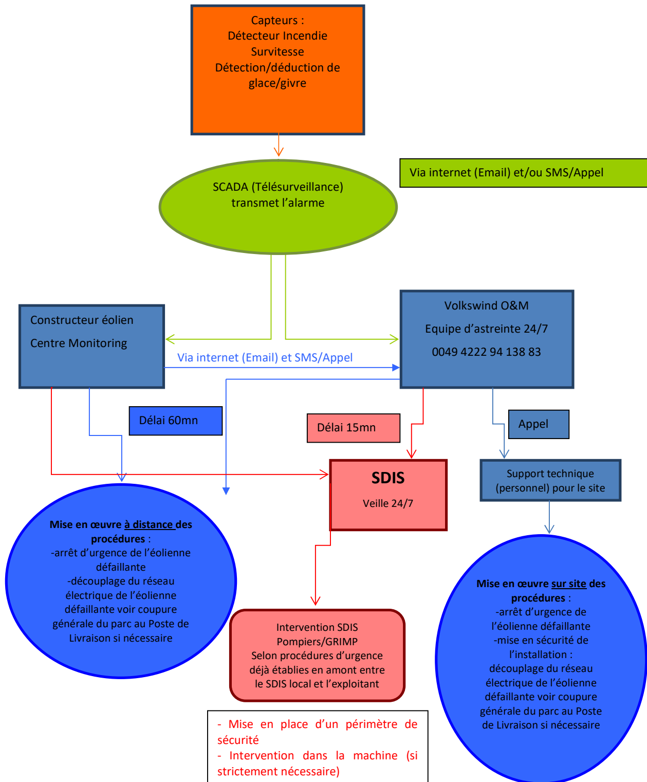
Figure 12 : Procédure en cas d'incident
