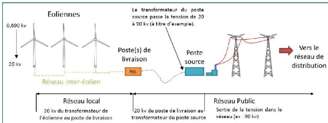
Figure 8 : Schéma de raccordement électrique d'un parc éolien
