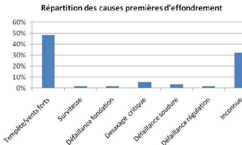
Figure 15 : Répartition des causes premières d'effondrement
