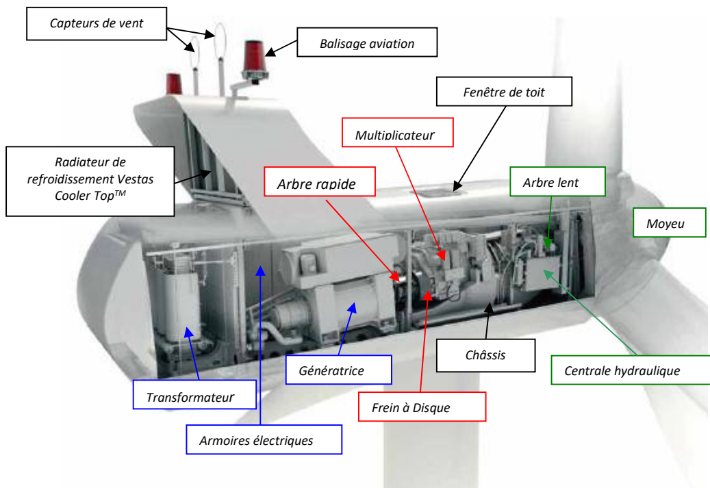
Figure 3 : Schéma technique de la nacelle Vestas
