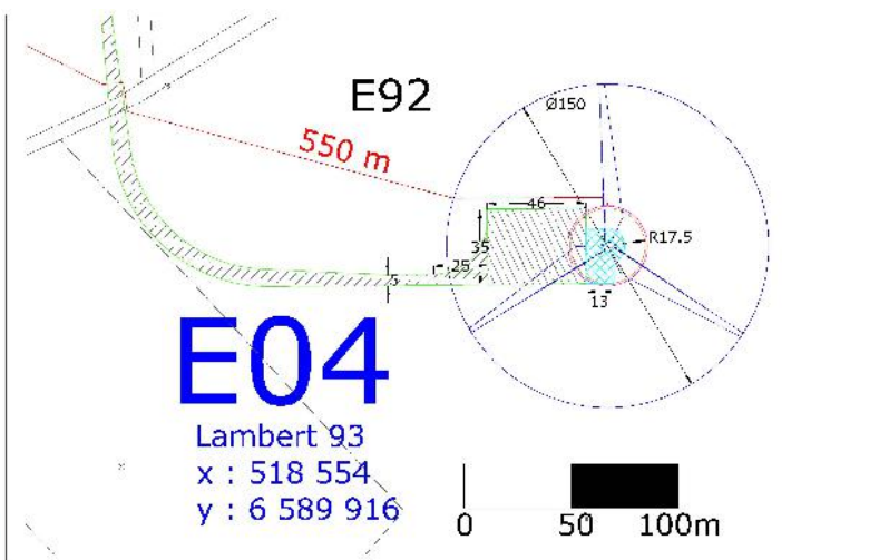
Figure 7 : Aires de montage et d'entretien des éoliennes
