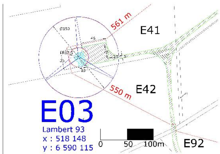
Figure 7 : Aires de montage et d'entretien des éoliennes
