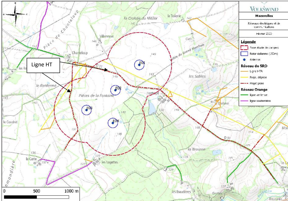
Carte 16 : Réseaux électriques et de communication
