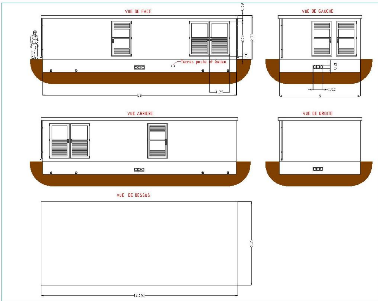
Figure 9 : Schéma d'un poste de livraison (12*5m)
