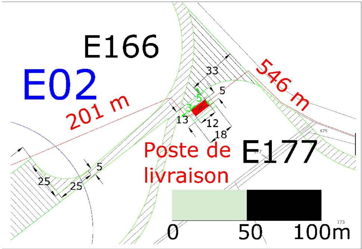
Carte 29 : Plan d'installation du poste de livraison
