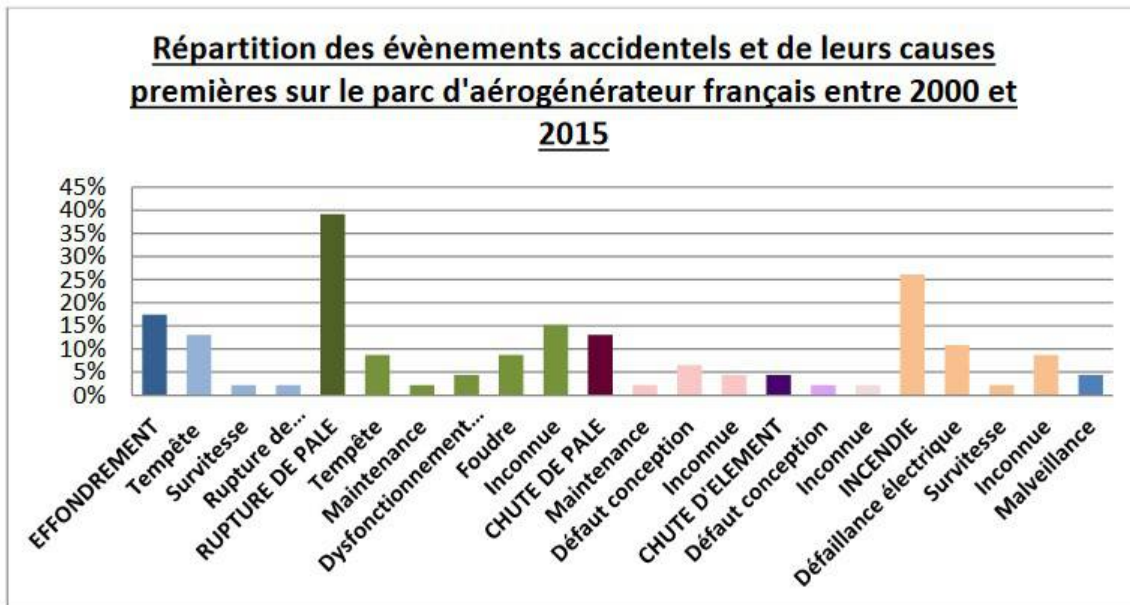
Figure 13 : Répartition des événements accidentels en France
