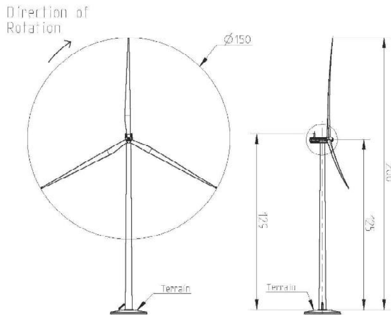
Figure 4 : Dessin d'élevation de l'éolienne Vestas V150- 4,2MW
