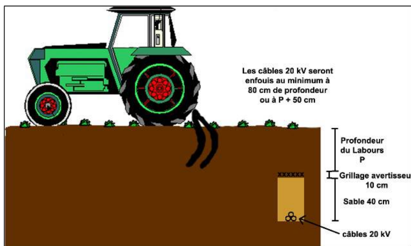
Figure 8 : Exemple de tranchées sous champs labouré
